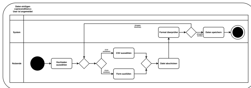
Abbildung 4.9: Daten einfügen
