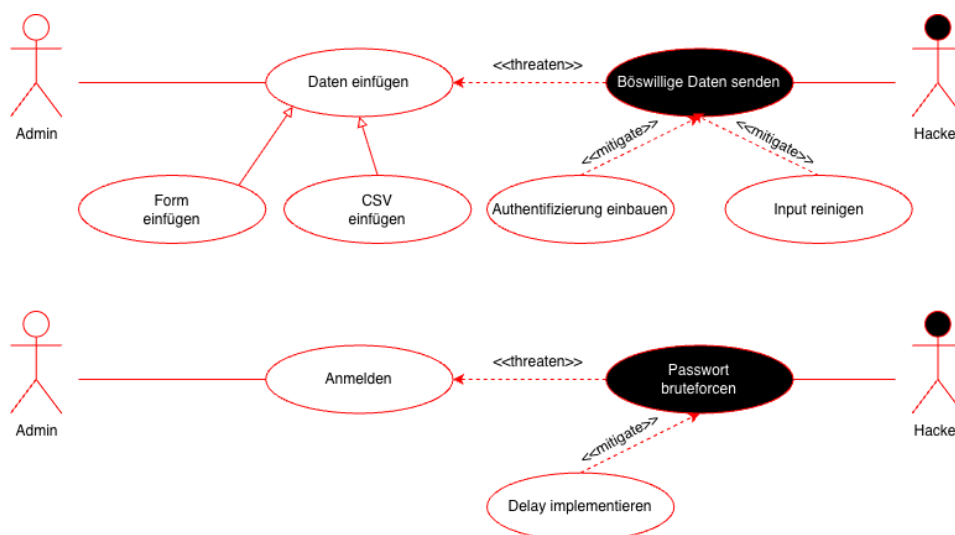
Abbildung 3.5: Misuse-Case-Diagramm
