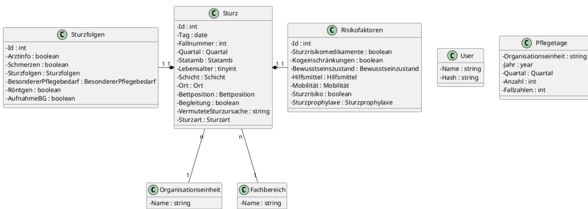
Abbildung 4.11: Klassendiagramm
